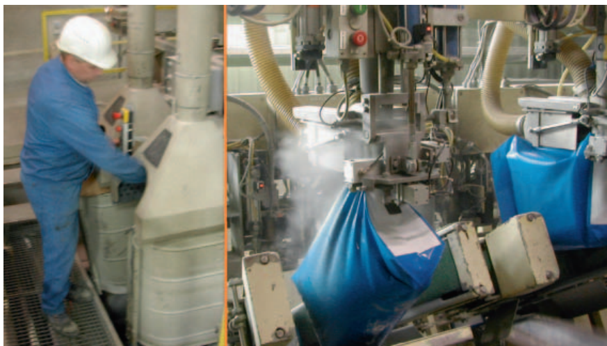
Im Vergleich: Wirksame (li) und trotz moderner Technik unzureichend optimierte Sackbefüllung (re)
