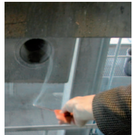
Ein am Absaugrohr angebrachter Flansch verbessert die Absaugwirkung erheblich.
