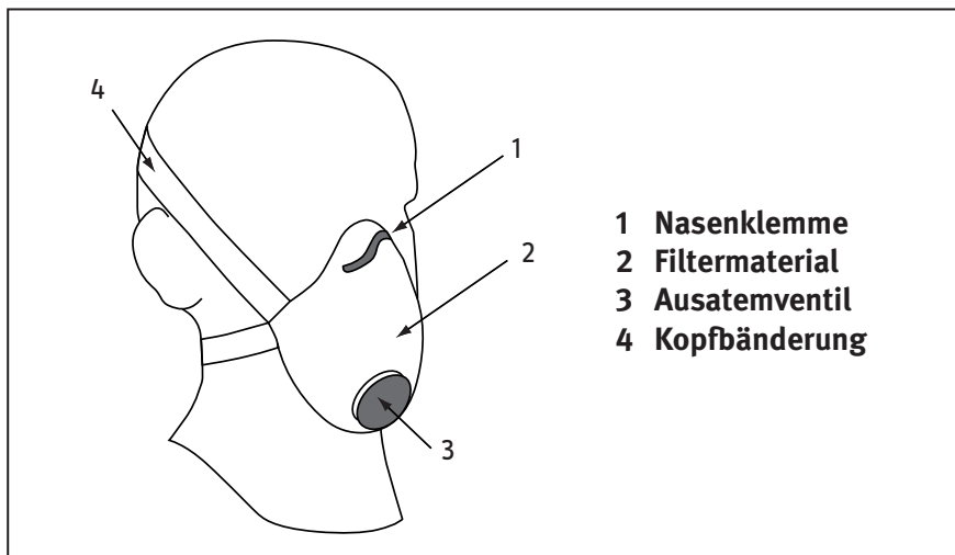
Partikelfiltrierende Halbmaske mit Ausatemventil und Nasenklemme
